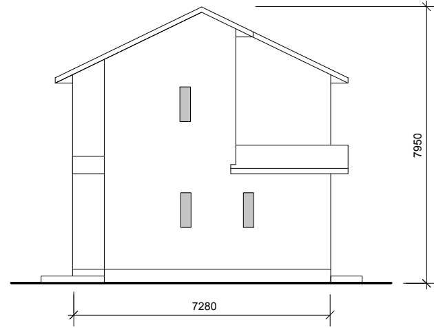
北立面図
