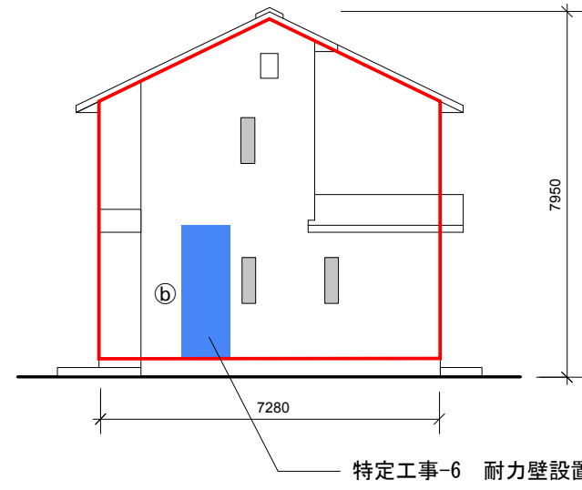
北立面図
