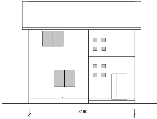
東立面図
