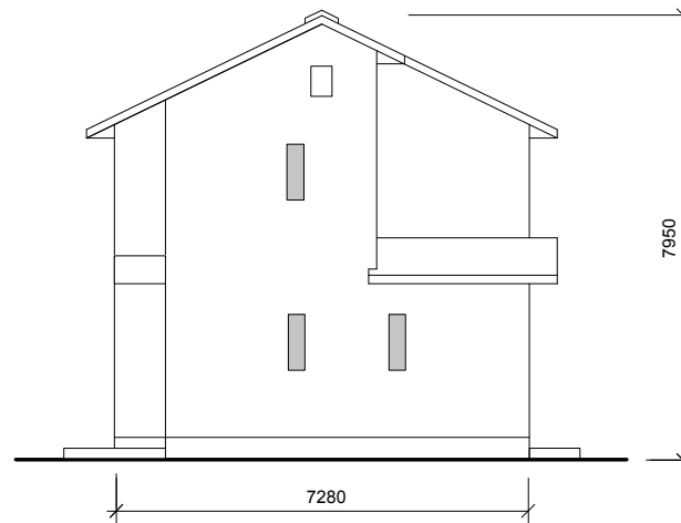
北立面図
