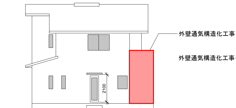
西立面図
