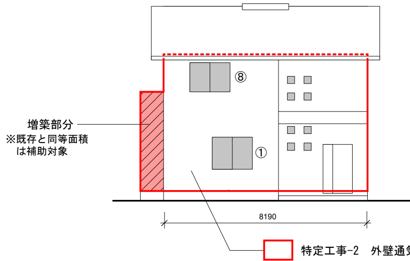
東立面図
